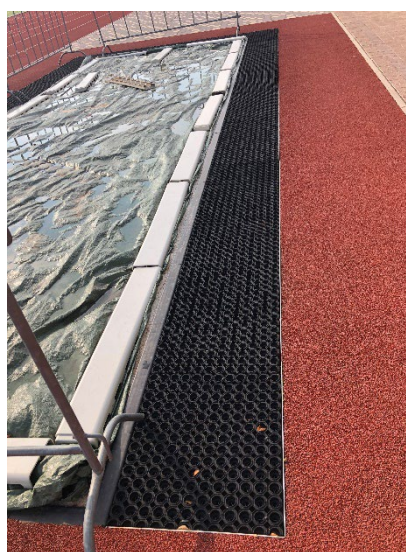
Tāllekšanas bedre – ACO Sport 7100 + ACO Sport 7400
