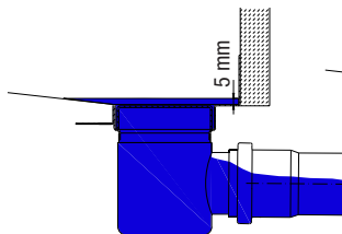
Uzstādīšana pie sienas (ūdens līmenis 5mm)
