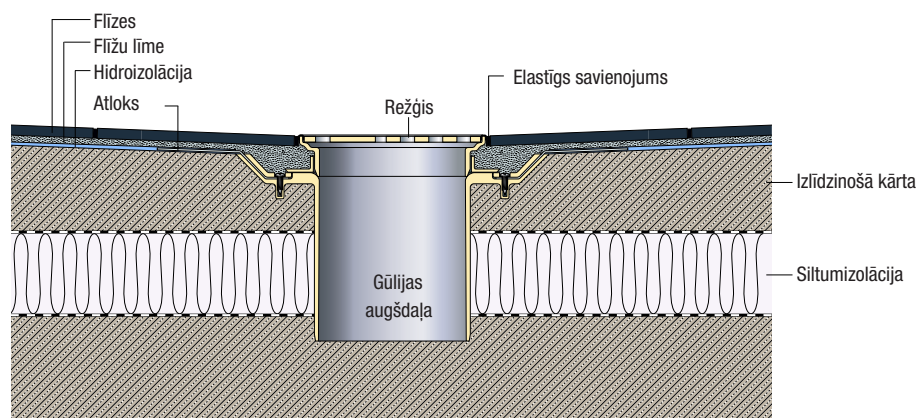
Gūlījas augšdaļa ar siltumizolāciju
