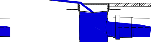
Uzstādīšana pie ieejas (bez ūdens uzkrāšanās)
