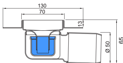
Pazemināta kanāla izmērs (konstrukcijas augstums 65 mm)
