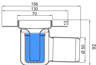
Standarta kanāla izmērs (konstrukcijas augstums 92 mm)
