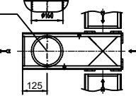
Sagatave izvadam Ø160
