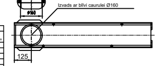
Kanāls L-1m ar izvadu Ø160
