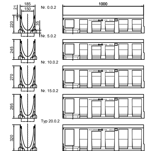
Kanāls L-1m ar izvadu Ø160
